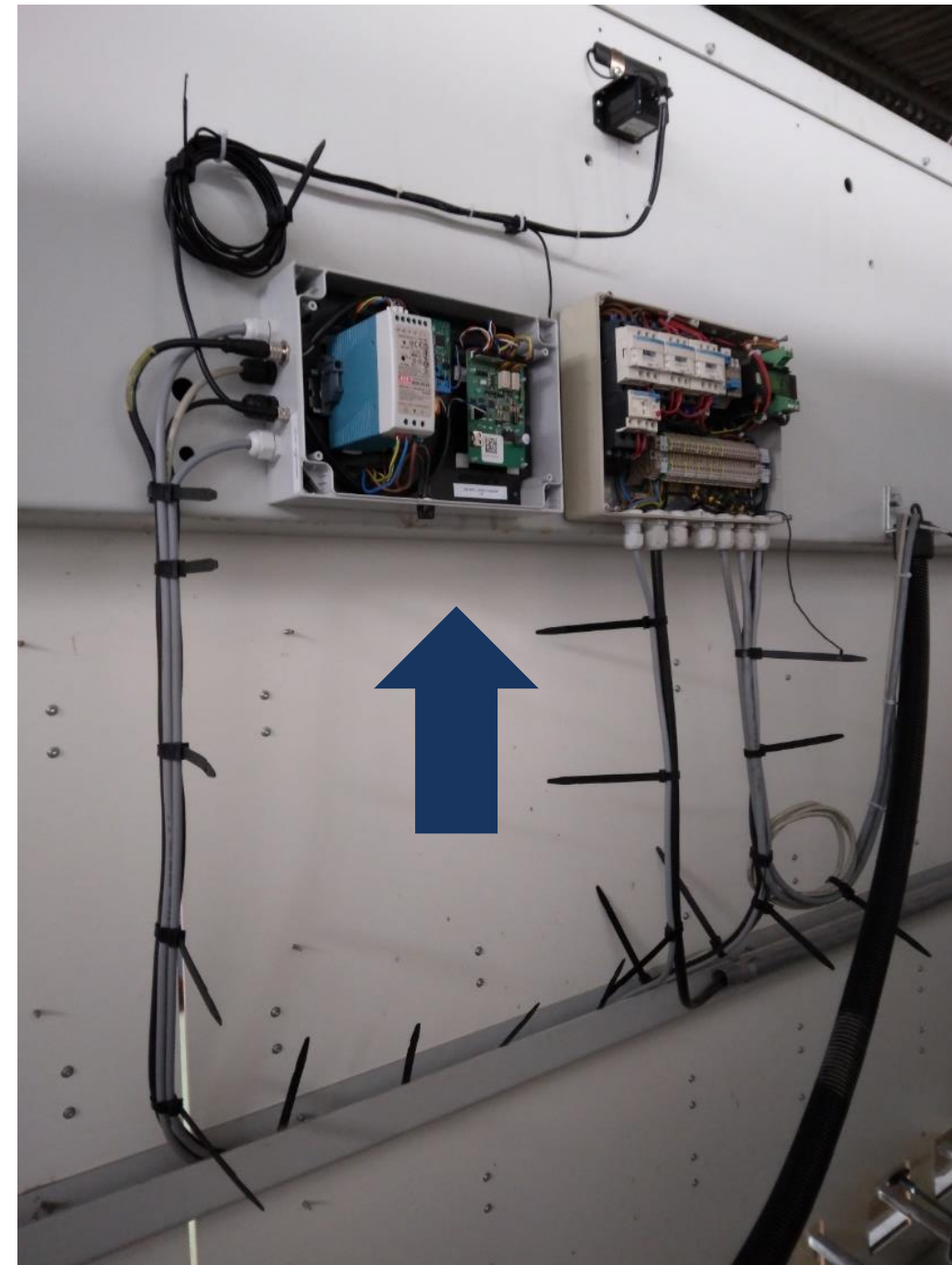
'Control Box' déportée à l'arrière de la scie (partie câblage).
