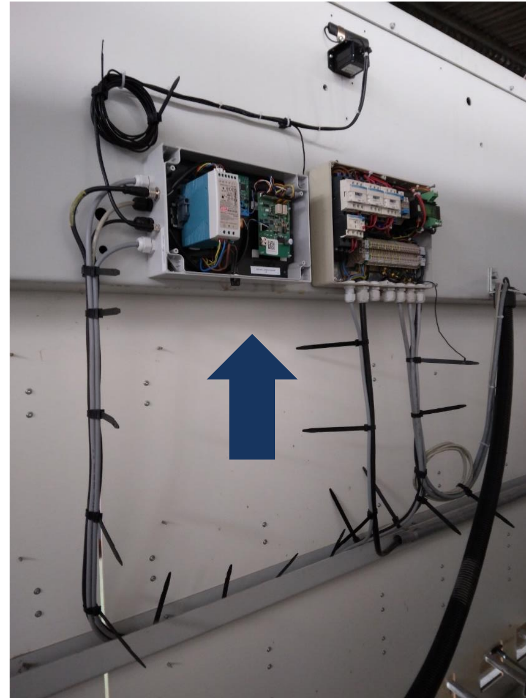
'Control Box' gedeporteerd naar de achterkant van de zaag (bedradingsgedeelte).
